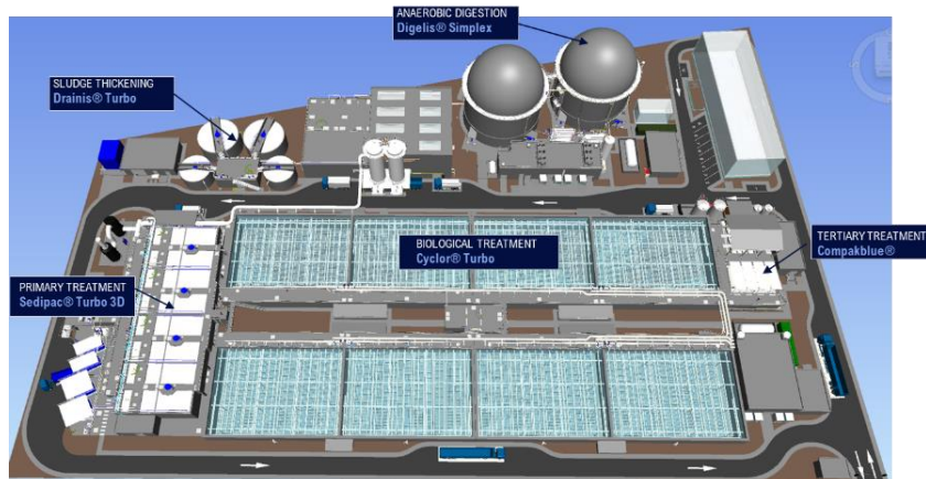
马尼拉中央污水处理系统的3D设计图，项目将使用苏伊士的前沿技术。
